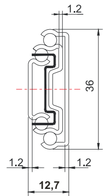
Profil-Schnitt
